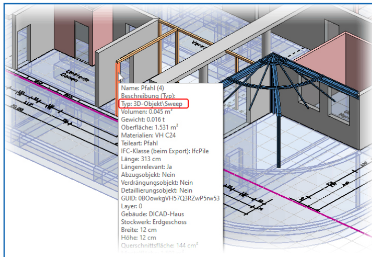
Abbildung 2: Ein Sweep-Objekt
