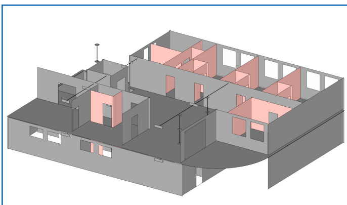
Abbildung 10: Unverbundene Bauteile
